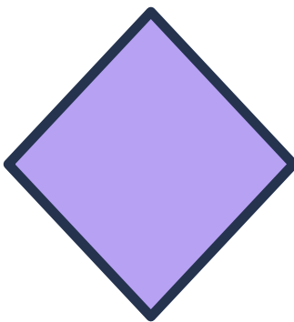
rhombus
